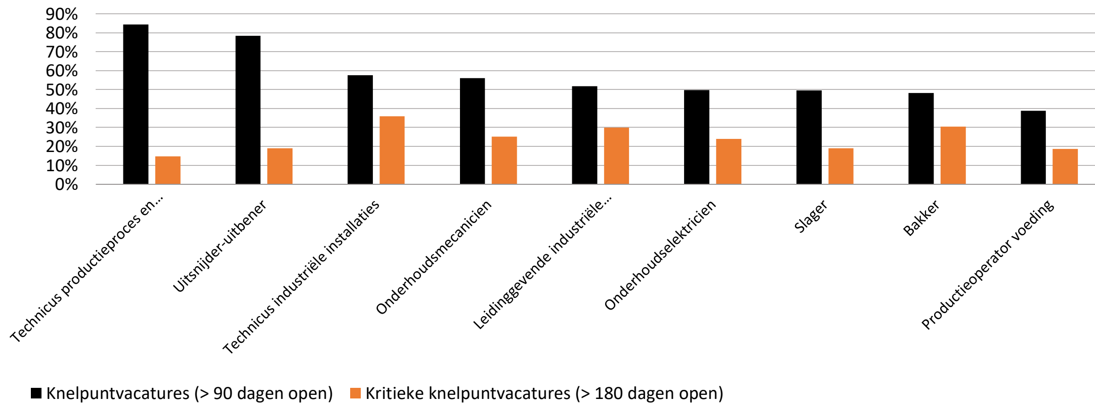
Aandeel knelpuntvacatures per type vacature in Vlaanderen
